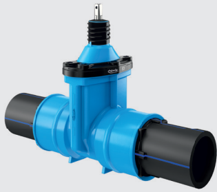
405-00 Gate valve „E3“ with PE fusion ends
